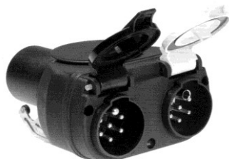
Art. 07.1037 Adattatore con spina 15 poli N°1 presa 7 poli "N"-N°1 presa 7 poli "S"
