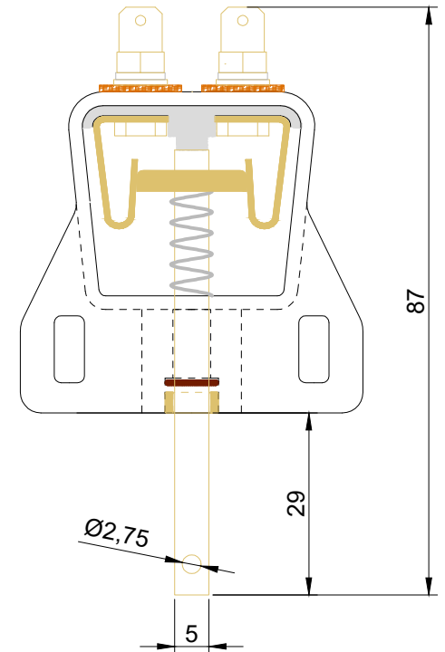
Art. 08.0802 Interruttore NC
