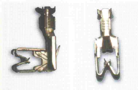
07.0480 sez. cavo 0,5-1,5
