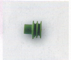
07.3070/V cavo 0,5-1,5 mm
